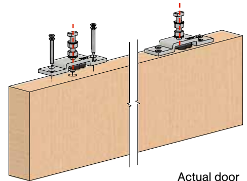
Actual door
