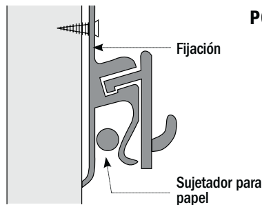
Riel de aluminio anodizado P6 Otros acabados se encuentran disponibles bajo pedido.
