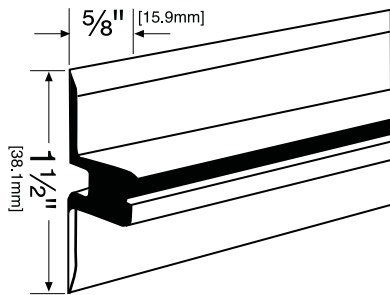
Riel de aluminio P5 con acabado natural
