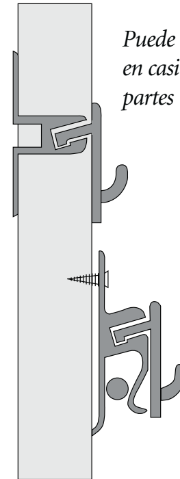
Riel de aluminio anodizado P6 Otros acabados se encuentran disponibles bajo pedido.
