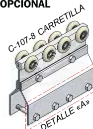
DETALLE "A" DE LA UBICACIÓN DE LOS ORIFICIOS DE LA CARRETILLA C-107-8 ANCHO TOTAL DE LA CARRETILLA: 7"
