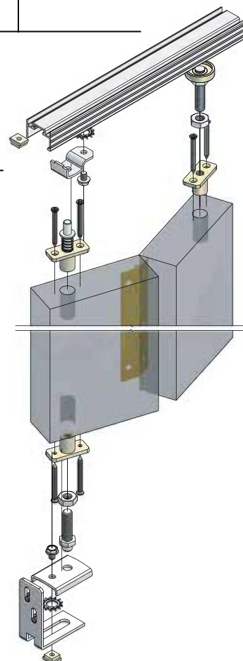
C-118 Panel (Para más detalles, ver página 67).
