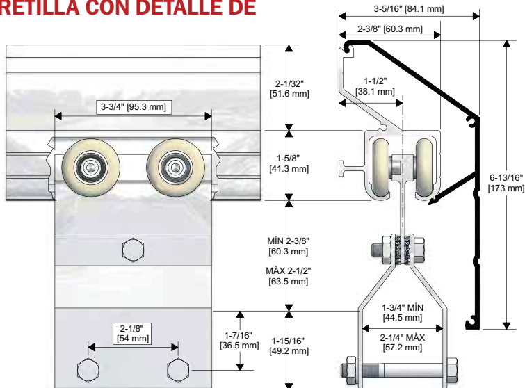
DETALLE "A" DE LA UBICACIÓN DE LOS ORIFICIOS DE LA CARRETILLA C-107-8 ANCHO TOTAL DE LA CARRETILLA: 7"
