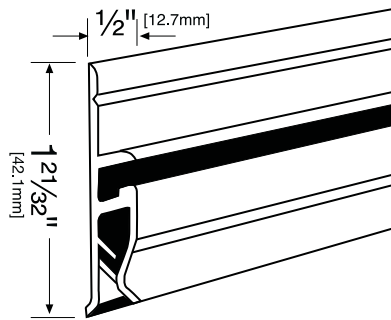
Riel de aluminio anodizado P6 Otros acabados se encuentran disponibles bajo pedido.
