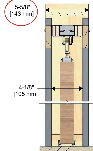
ESQUEMA DEL EQUIPO DE PUERTAS CORREDIZAS PARA PAREDES DE 2" X 6"
