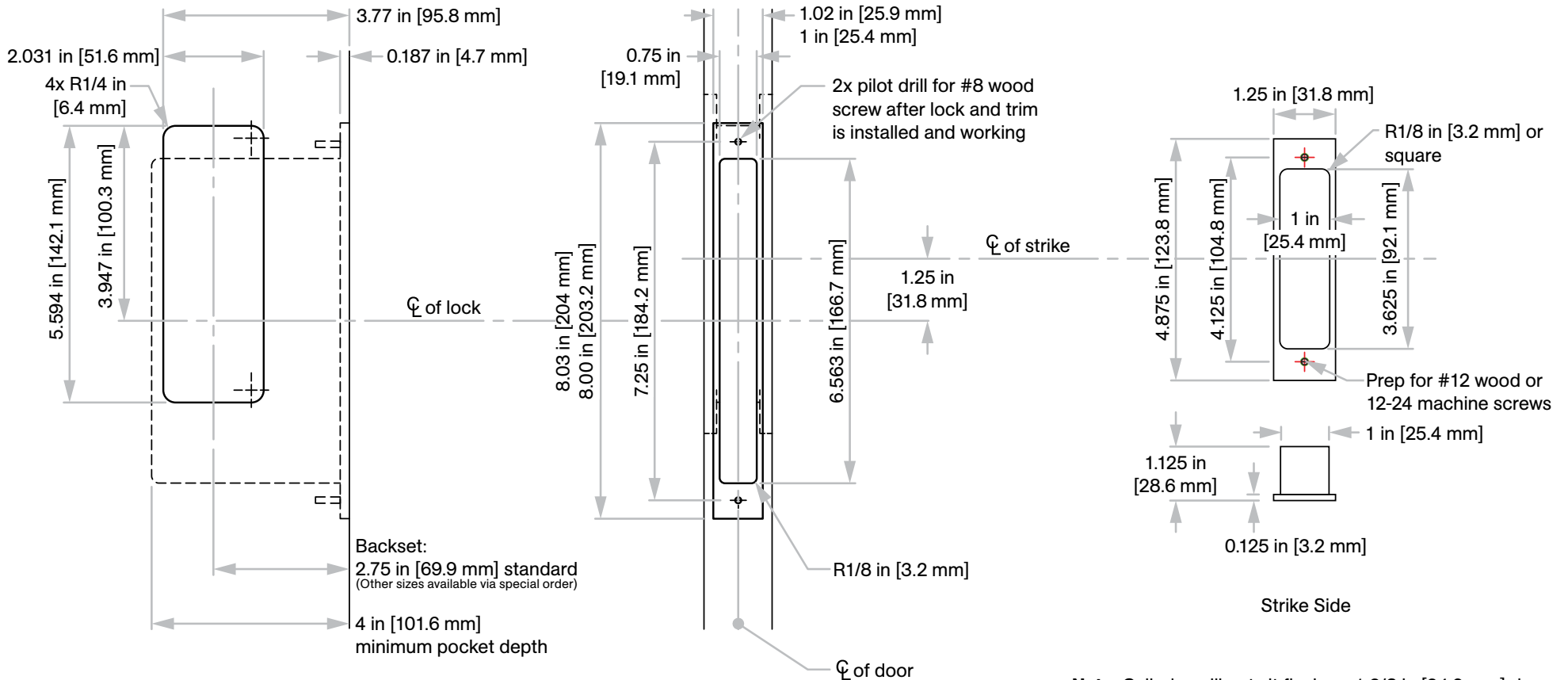
C-90L Lock and Edge Pull Body
