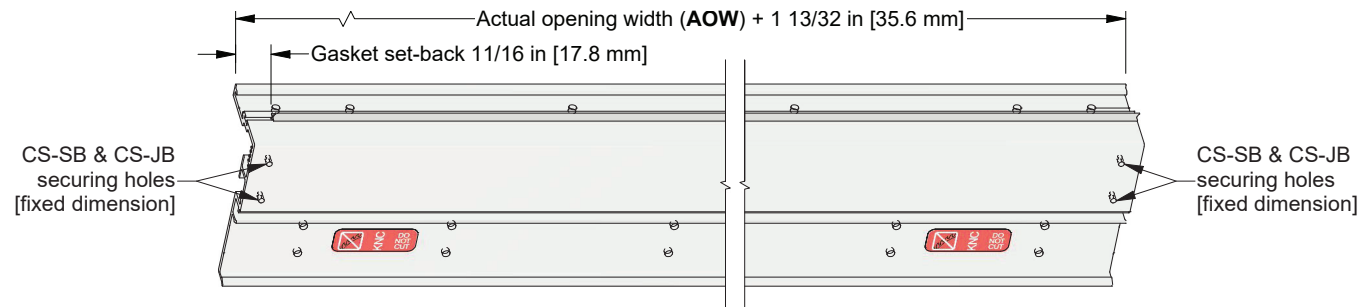
CS-HB Header Base (1)
