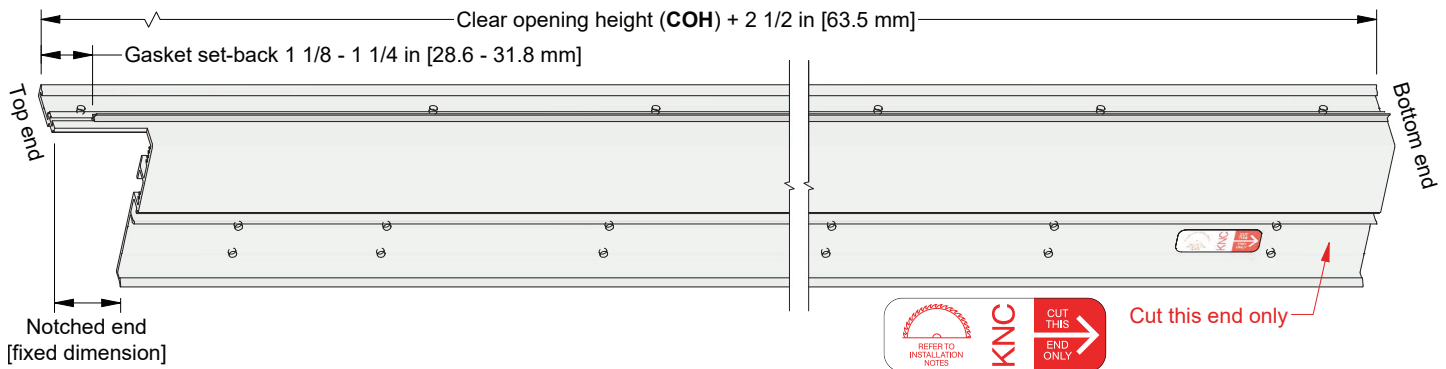
CS-JB Jamb Base (1)
