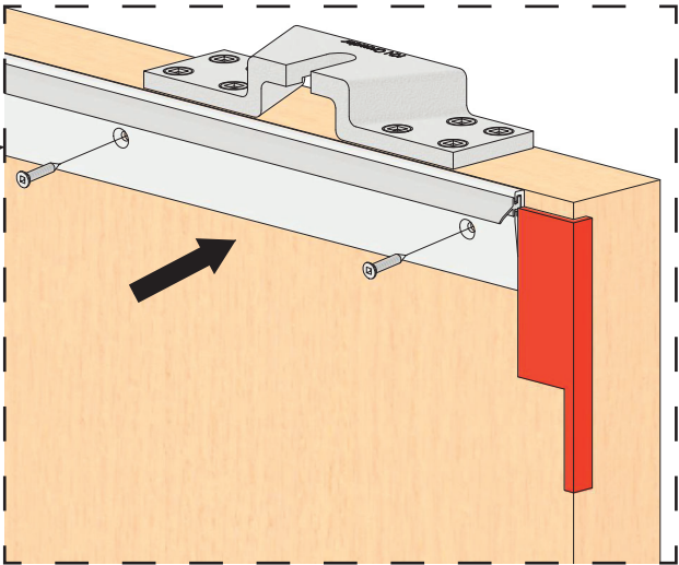
CS-DRT Door Template Tool Set (1)
